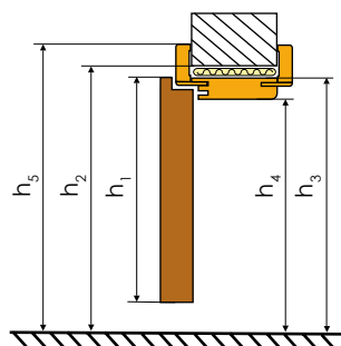
WYMIARY OŚCIEŻNICY REGULOWANEJ I SKRZYDŁA (mm)
