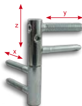
zawias wkręcany z regulacją 3-D
